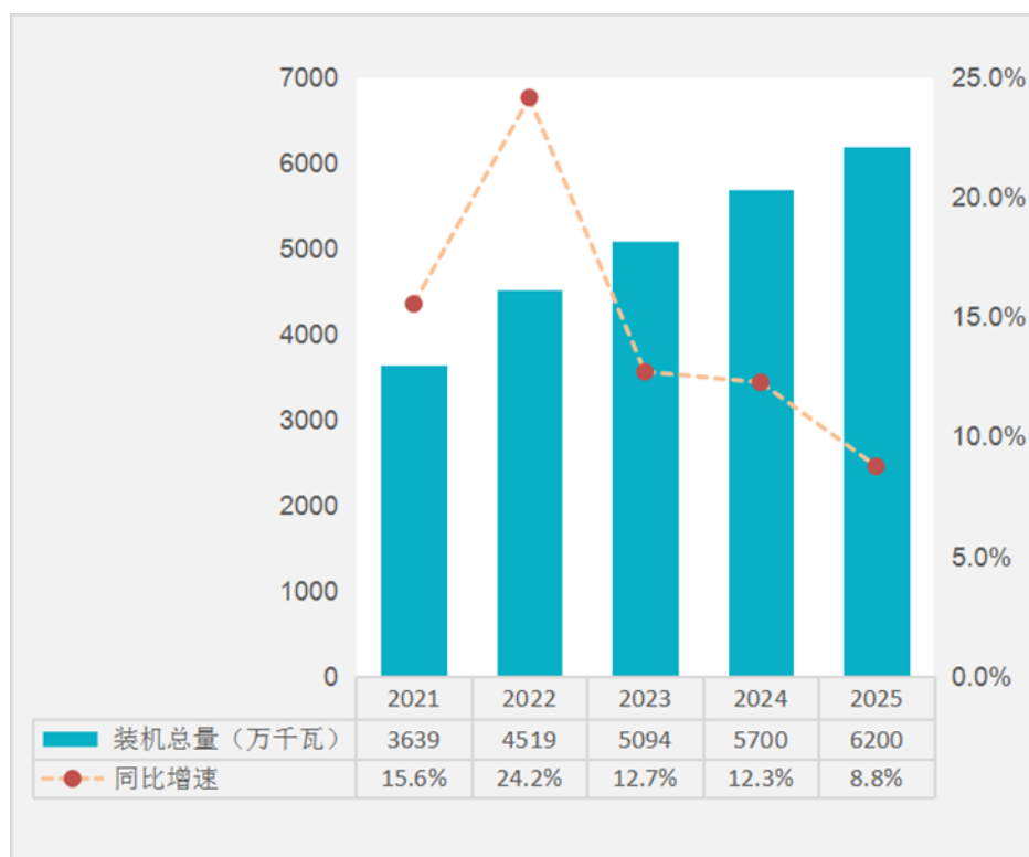
图表：2021-2025 年中国抽水蓄能装机总量分析
